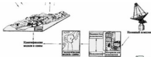
Рисунок 1 – схема системы дистанционного зондирования
